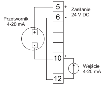
Rys. 4c - Podłączenie 4÷20 mA z zasilaniem pętli
