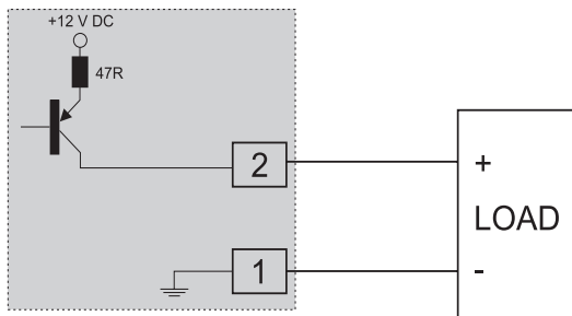
Rys. 5 - Wyjście analogowe I/O5.
