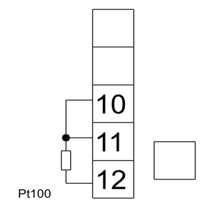
Rys. 3b - Wejście Pt100
