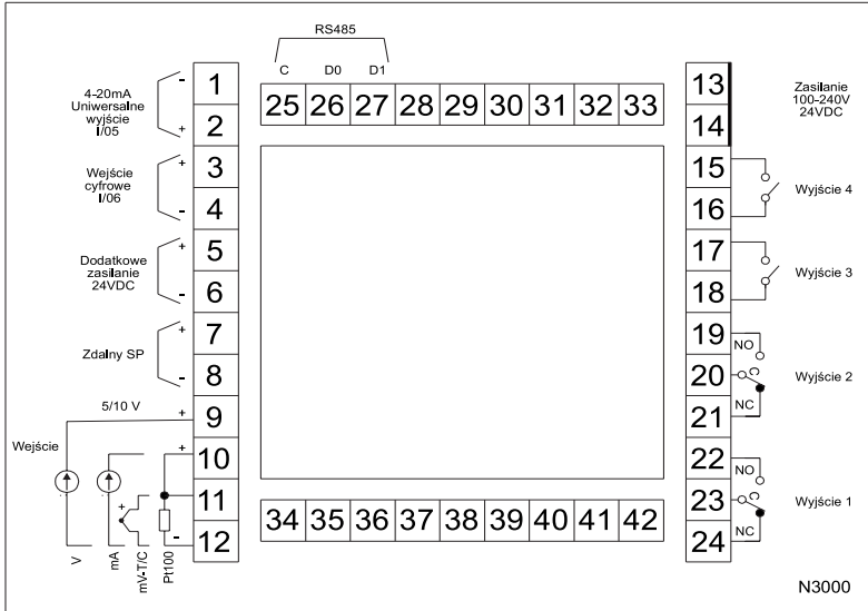
Rys. 1 - Schemat elektryczny regulatora
