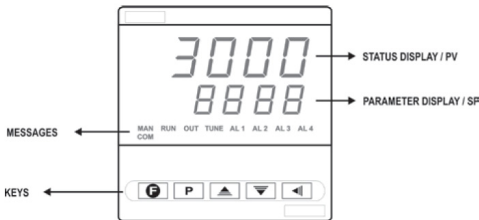
Rys. 8 - Panel przedni regulatora N3000
