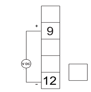
Rys. 4b - Podłączenie 5 V/10 V
