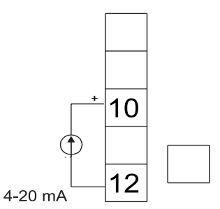
Rys. 4a - Podłączenie 4÷20 mA
