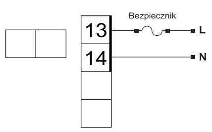
Rys. 2 - Podłączenie napięcia zasilającego
