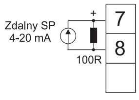
Rys. 4d - Zdalny SP 4÷20mA
