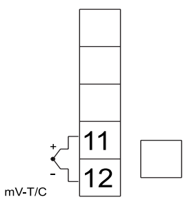
Rys. 3a - Wejście TC
